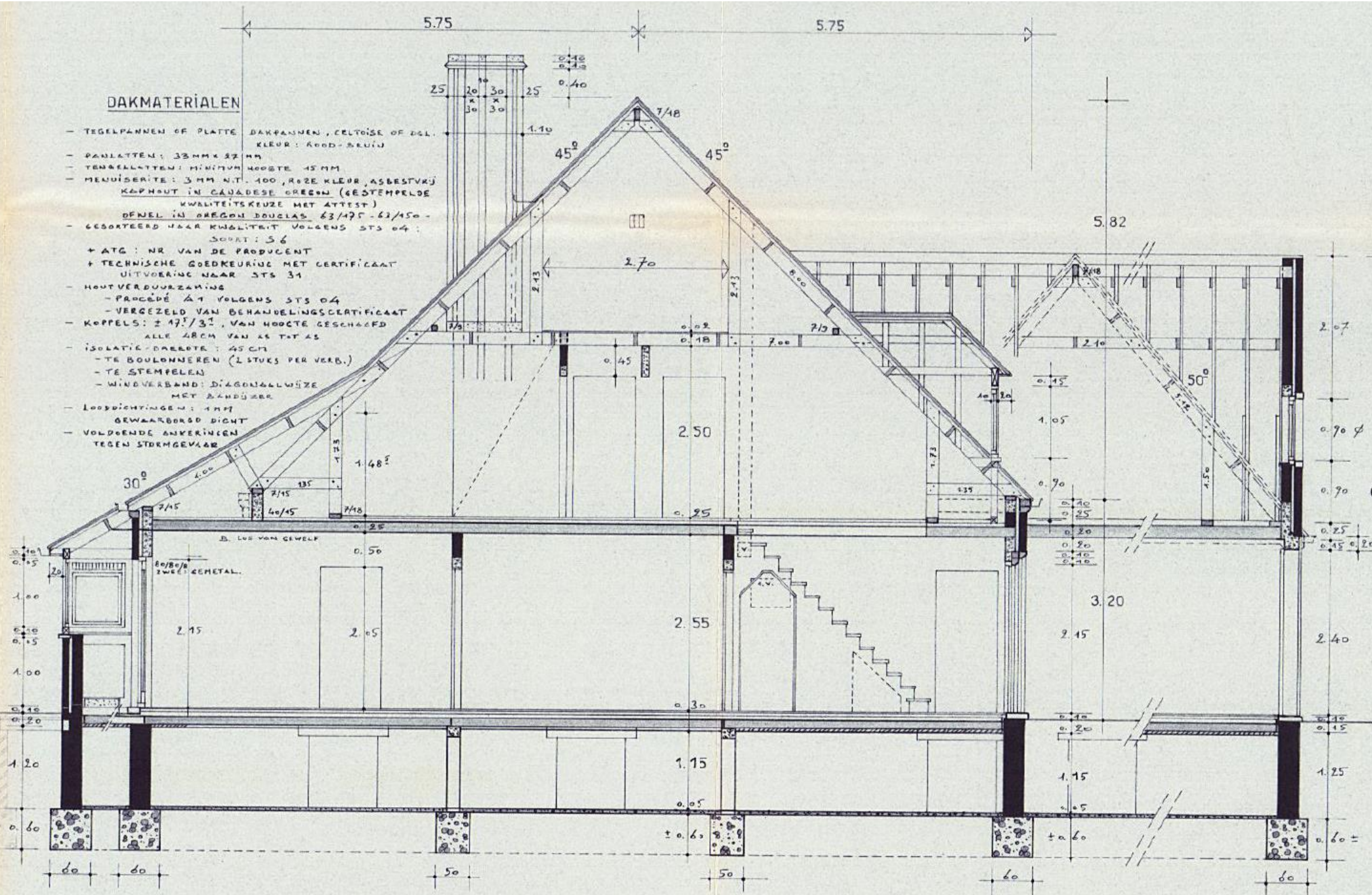
DWARSDOORSNEDE
